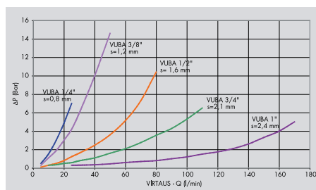
Painehäviökäyrä
