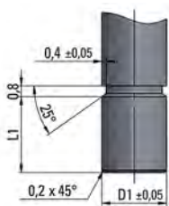
Putkijatkeen uran mitoitus
