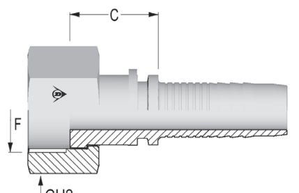
SISÄKIERRE BSP (HIAB) A50003-XX-XX
