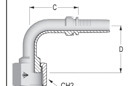
90° SISÄKIERRE ORFS M50A28-XX-XX
