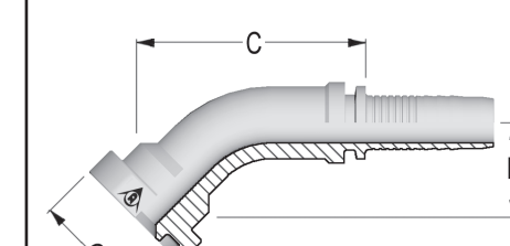
45° LAIPPALIITIN SAE 6000 PSI 501610-XX-XX
