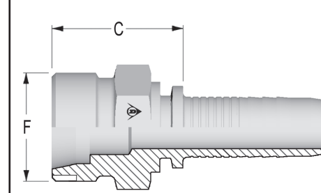
PUTKITARTUNNAT RASKAS SARJA CES - DIN 3853 501700-XX-XX
