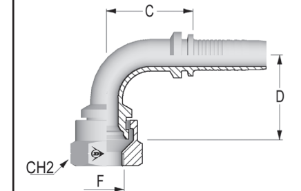
90° SISÄKIERRE JIS 60° (MITSUBISHI) A50A06-XX-XX
