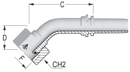
45° SISÄKIERRE BSP 60° A50061-XX-XX
