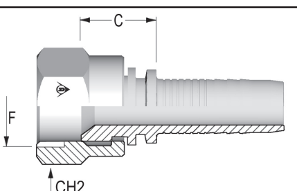
SISÄKIERRE JIC 37° A50005-XX-XX
