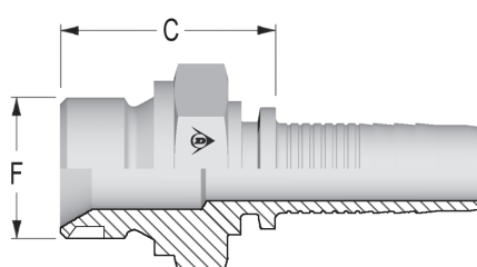
ULKOKIERRE BSP 60° 500120-XX-XX
