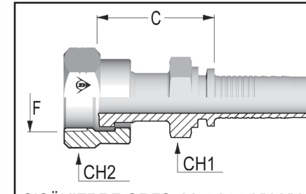
SISÄKIERRE ORFS M50A26-XX-XX
