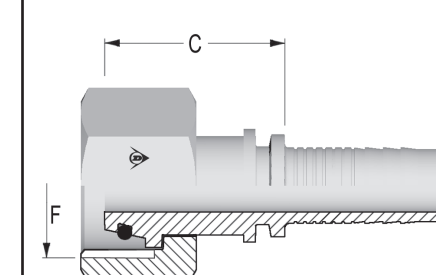
SISÄKIERRE DKOS - DIN 3865 A50179-XX-XX
