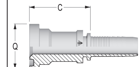
LAIPPALIITIN SAE 3000 PSI 500250-XX-XX
