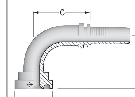
90° LAIPPALIITIN SAE 3000 PSI 500580-XX-XX
