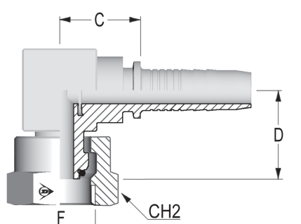
90° SISÄKIERRE BSP 60° A50180-XX-XX
