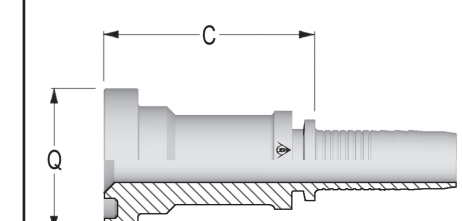
LAIPPALIITIN SAE 6000 PSI 501590-XX-XX
