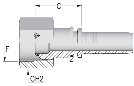
SISÄKIERRE BSP 60° A50001-XX-XX
