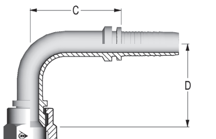
90° SISÄKIERRE JIC 37° A50054-XX-XX
