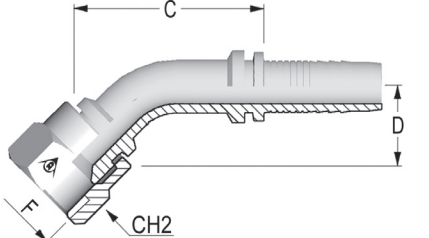
45° SISÄKIERRE JIC 37° A50064-XX-XX
