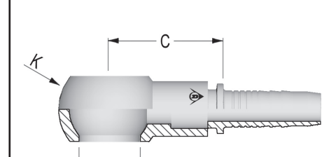
BANJOLIITIN M 500RLO-XX-XX
