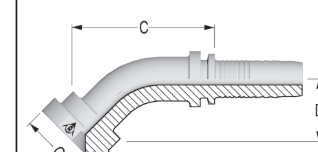
45° LAIPPALIITIN SAE 3000 PSI 500680-XX-XX
