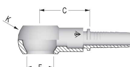
BSP BANJOLIITIN RNR 502190-XX-XX
