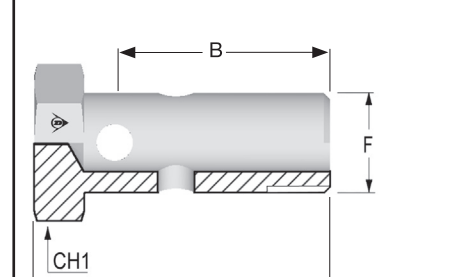
BANJOPULTTI M 570RPL-MXX
