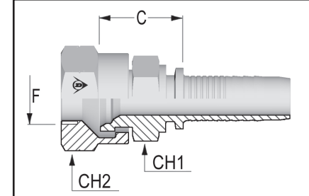
SISÄKIERRE JIS 60° (MITSUBISHI) A50A02-XX-XX
