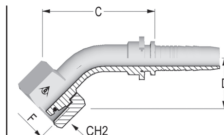
45° SISÄKIERRE DKOS - DIN 3865 A50A56-XX-XX
