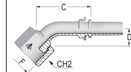
45° SISÄKIERRE ORFS M50A27-XX-XX
