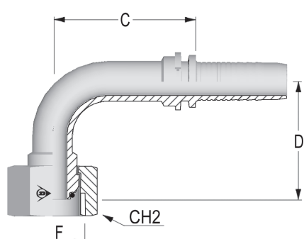
90° SISÄKIERRE BSP 60° A50051-XX-XX
