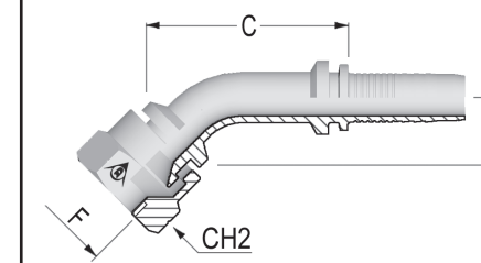
45° SISÄKIERRE JIS 60° (MITSUBISHI) A50A07-XX-XX
