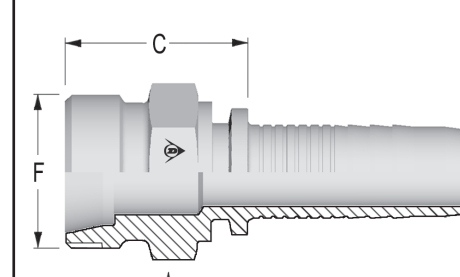
PUTKITARTUNNAT KEVYT SARJA CEL - DIN 3853 501690-XX-XX
