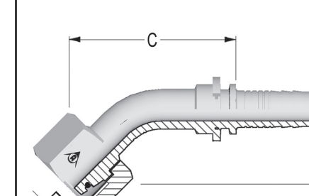
45° SISÄKIERRE DKOL - DIN 3865 A50A51-XX-XX
