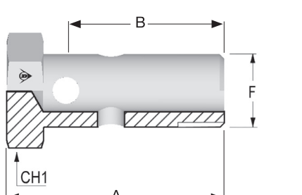
BSP BANJOPULTTI 570RPL-XX-XX
