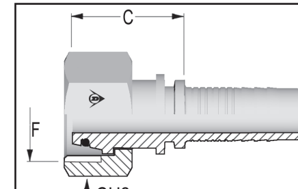
SISÄKIERRE DKOL - DIN 3865 A50146-XX-XX
