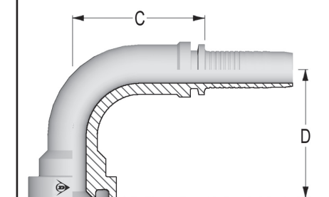
90° LAIPPALIITIN SAE 6000 PSI 501600-XX-XX
