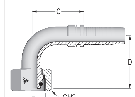
90° SISÄKIERRE DKOS - DIN 3865 A50A57-XX-XX
